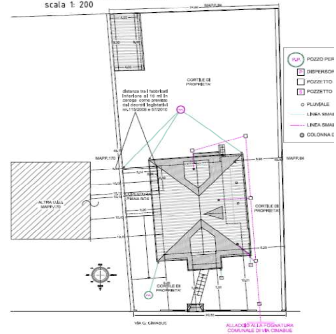
PLANIMETRIA GENERALE - SCHEMA FOGNATURA - SUP. COPERTA STATO ATTUALE DEI LUOGHI scala 1: 200
